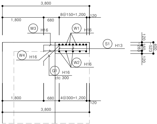
단면도(B-B) S=1:50
